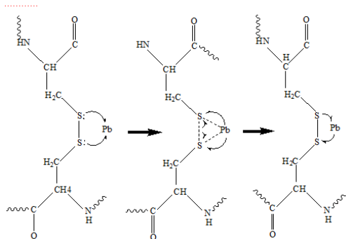
Gambar 6. Gugus sulfida pada asam amino sistein mengikat logam Pb
