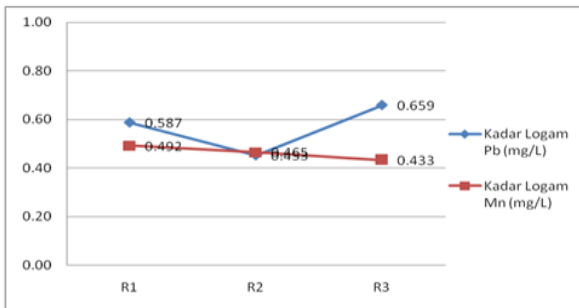
Gambar 1. Kadar logam Pb dan Mn pada udang windu di titik 1
