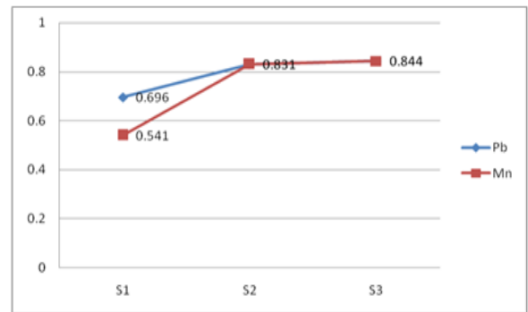
Gambar 2. Kadar logam Pb dan Mn pada udang windu di titik 2
