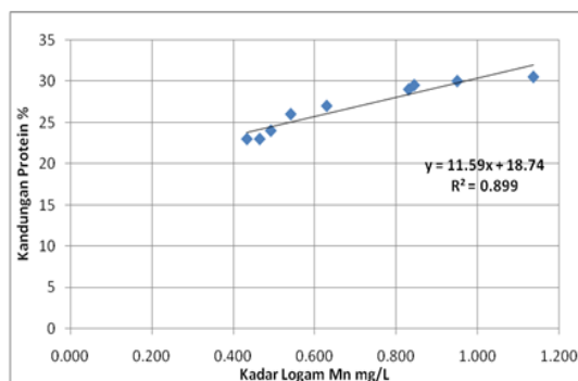
Gambar 5. Korelasi kadar logam Mn dan kandungan protein
