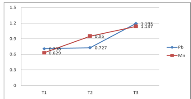
Gambar 3. Kadar logam Pb dan Mn pada udang windu di titik 3
