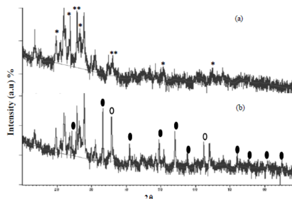
Gambar 3. Hasil analisa XRD (a) zeolit setelah aktivasi dan (b) zeolit-Fe 2 O 3
